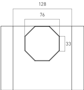
Vista inferior
